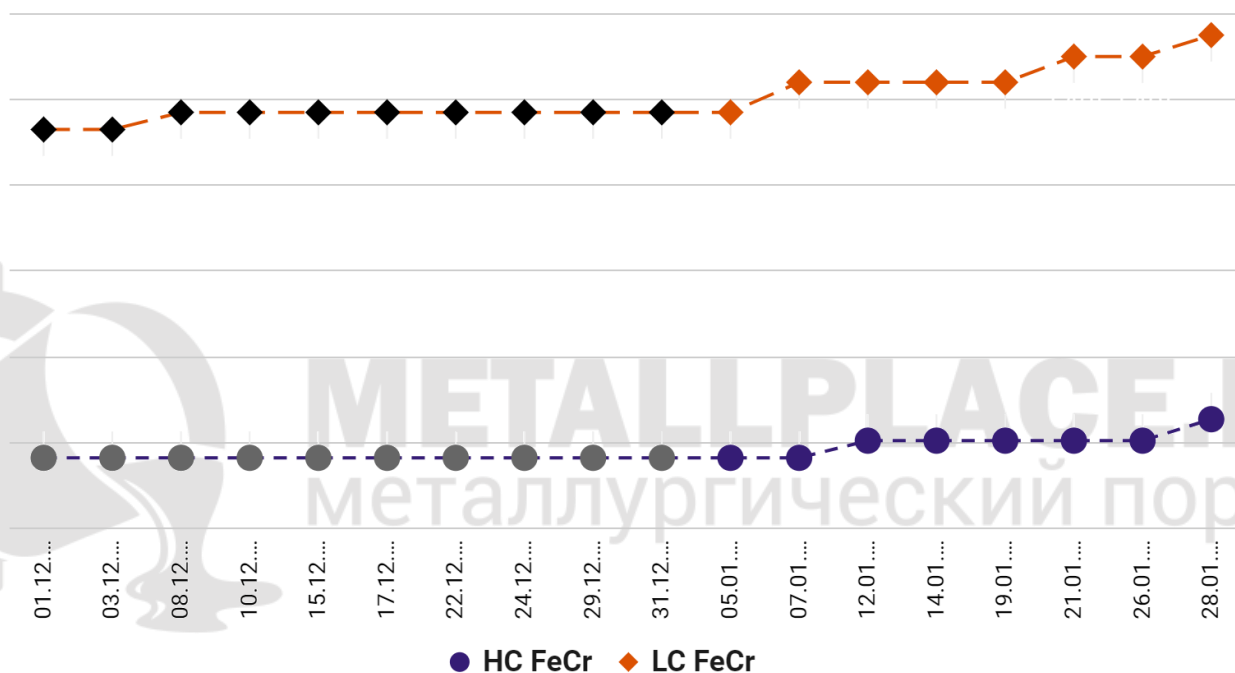
Цена на феррохром, USD/фунт Cr DDP Европа
